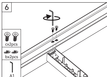
Lampenhalter mit Schrauben befestigen.
