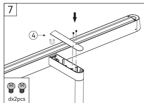
Abdeckung magnetisch anbringen.
