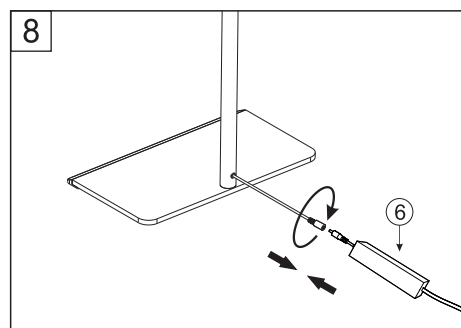
Netzteilkabel mit dem Lichtrohr verbinden und um 90° drehen.
