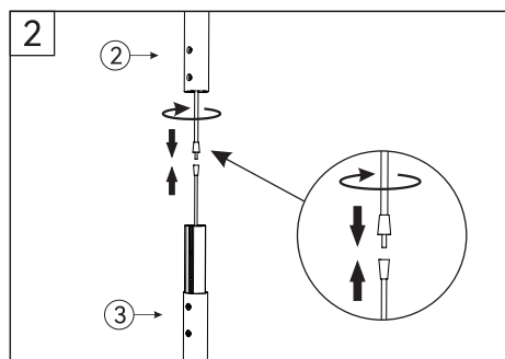
Netzkabel in der Lampenstange verbinden und um 90° drehen.
