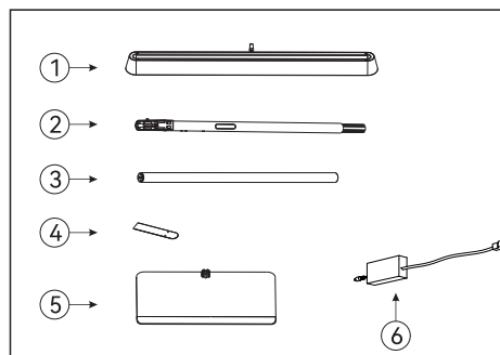
Produktübersicht: ①Lampenkopf ②Obere Lampenstange ③Untere Lampenstange ④Abdeckungen ⑤Bodenplatte ⑥Netzteil
