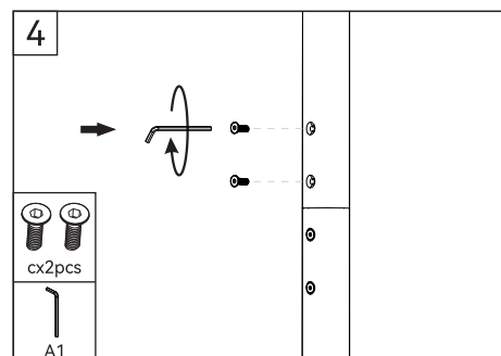
Lampenstange befestigen.
