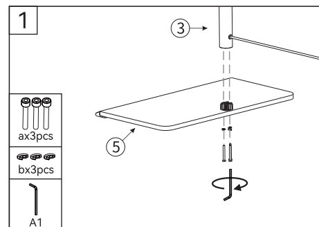
Lampenstange an der Bodenplatte befestigen.
