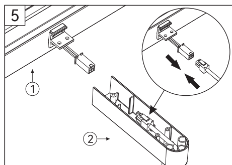
Anschlussklemme verbinden.
